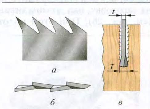
Рис. 25. Зубья пилы для продольного пиления: a – форма зубьев; б – вид разведённых зубьев; в – процесс пиления (вид со стороны пласти заготовки)
