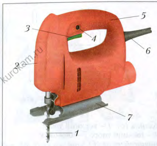
Рис. 30. Электроробзик: 1 – пилка; 2 – корпус; 3 – кнопка включения; 4 – кнопка блокировки включения; 5 – ручка; 6 – электрический шнур; 7 – опора
