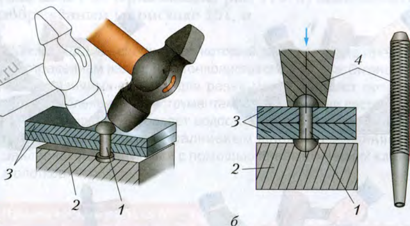
Рис. 148. Формирование головки заклёпки:
