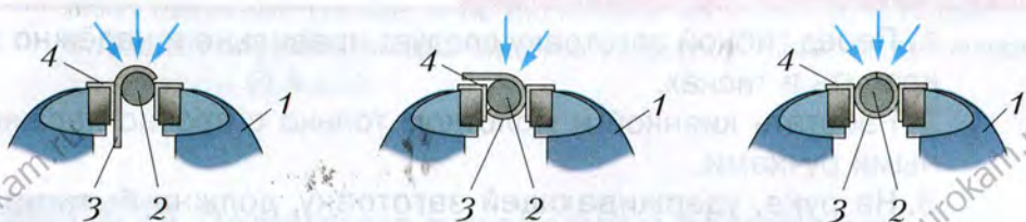
Рис. 131. Гибка проволочного кольца с помощью цилиндрической оправки: 1 – тиски; 2 – цилиндрическая оправка; 3 – заготовка; 4 – уголки
