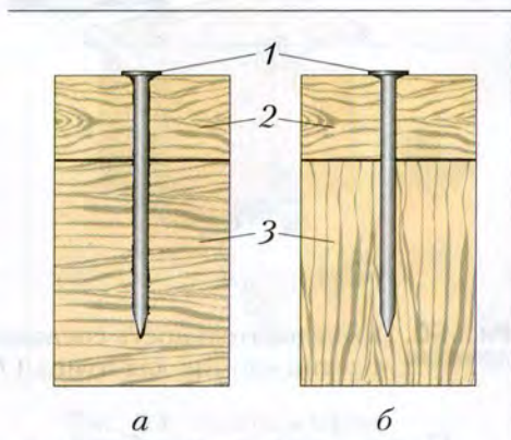
Рис. 49. Соединение деталей гвоздями: а – поперёк волокон; б – вдоль волокон основной детали (показано в разрезе): 1 – гвоздь; 2 – прибиваемая деталь; 3 – основная деталь
