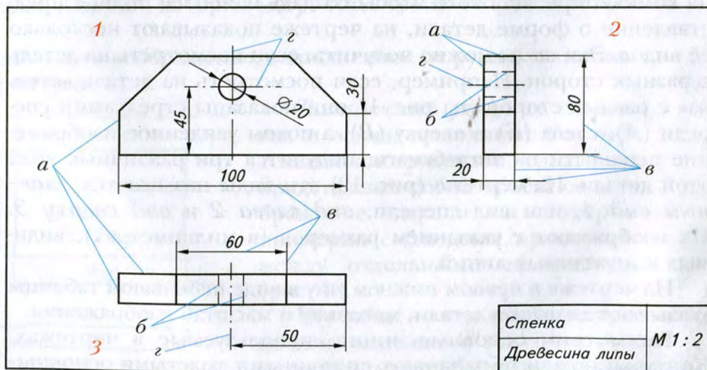
Рис. 12. Чертёж детали «стенка»: 1 – главный вид; 2 – вид слева; 3 – вид сверху: а – основные линии; б – штриховые линии; в – размерные и выносные линии; z – штрихпунктирные линии
