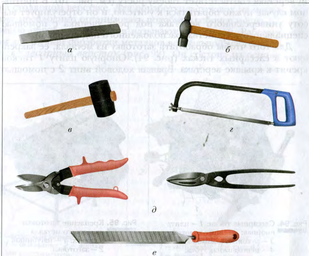
Рис. 96. Инструменты для ручной обработки тонколистового металла и проволоки: а – зубило; б – слесарный молоток; в – киянка; г – ножовка; д – ножницы по металлу; е – напильник
