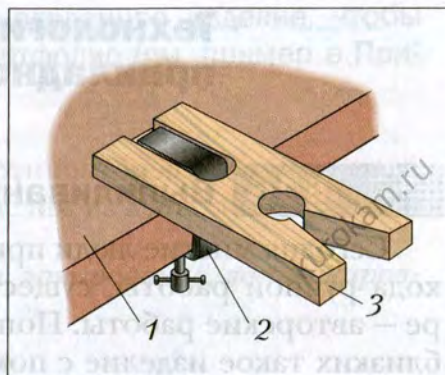
Рис. 70. Выпиловочный столик: 1 – верстак; 2 – струбина; 3 – дощечка
