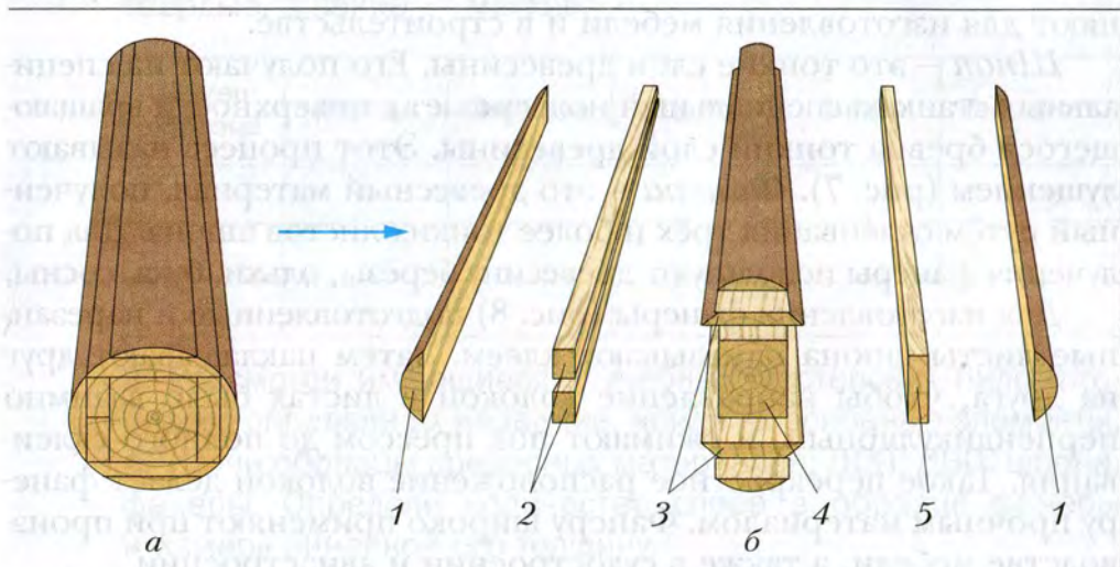
Рис. 5. Виды пиломатериалов: а – бревно с разметкой; б – виды пиломатериалов: 1 – горбыль; 2 – брус; 3 – доска необрезная; 4 – доска обрезная; 5 – доска обрезная
