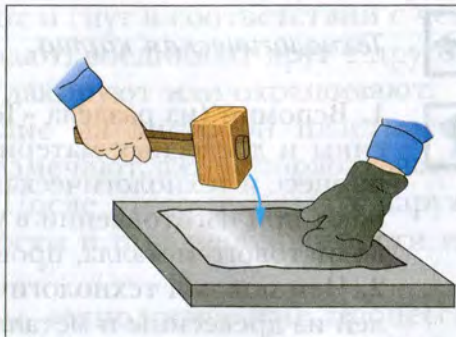
Рис. 105. Правка тонколистовой заготовки киянкой
