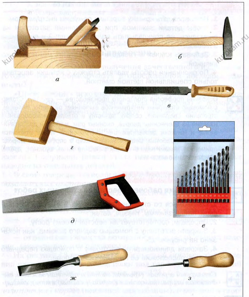
Рис. 17. Основные инструменты для обработки древесины: а – рубанок; б – молоток; в – напильник; г – киянка; д – ножовка; е – свёрла; ж – стамеска; з – шило
