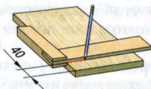
Рис. 20. Последовательность разметки детали из древесины (1–10)
