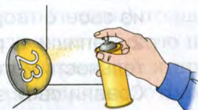
Рис. 103. Изготовление номерка на дверь квартиры (заготовка – оргстекло): a – общий вид (номер и места расположения крепёжных отверстий назначает ученик); б – технологический процесс (1–8)
