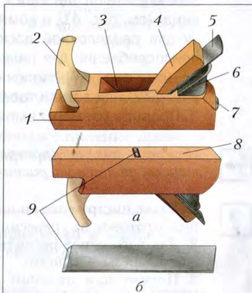
Рис. 33. Рубанок: а – общий вид;
